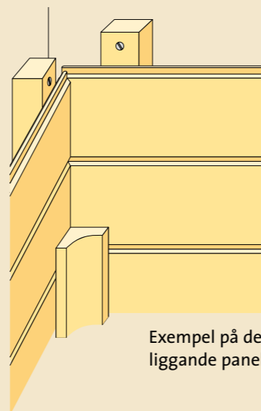
Avsluta panelen 10 från angränsande vägg.
