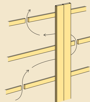
Takpanelen spikas eller skruvas i varje regel.
