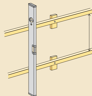
Spikläkt för ventilerad panel.
