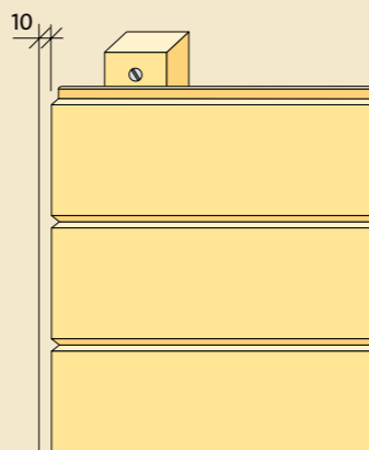
Avsluta panelen 10 från angränsande vägg.
